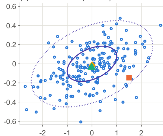
(d) R1: p_0 , LSM6DSV16X ( n = 100 )
